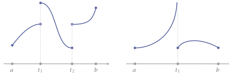
Abb 7 Stückweise, und nicht stückweise stetige Funktion
